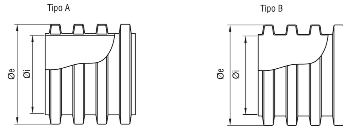
Tipo A : Perfil corrugado exterior y liso interior
