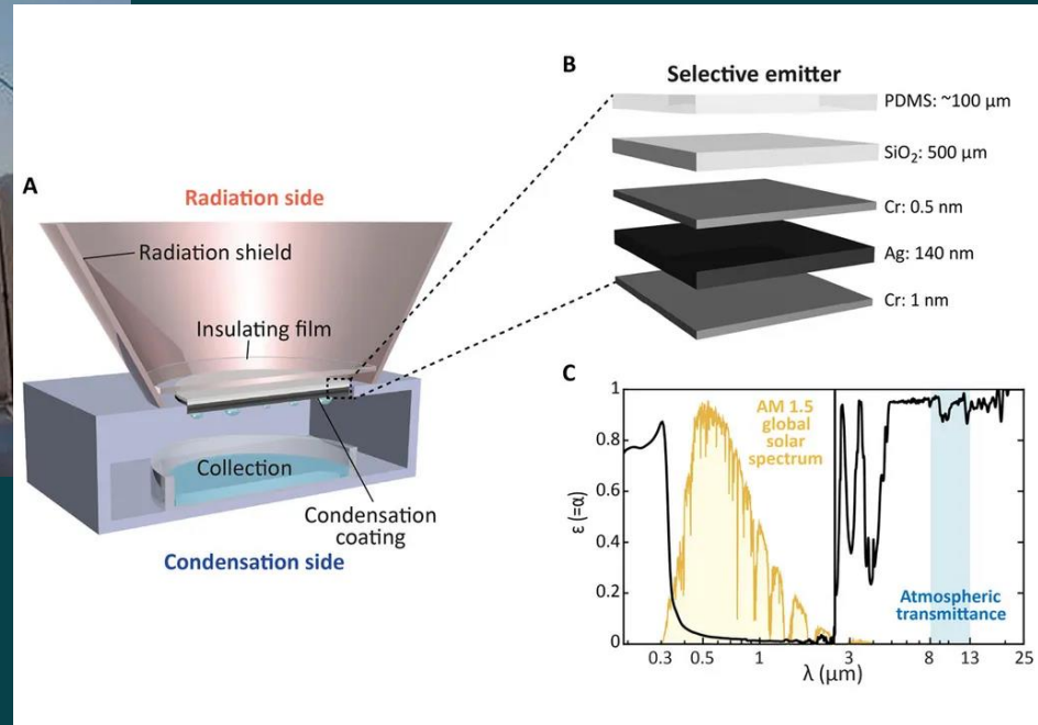
CONDENSADOR DE AGUA DE LA ATMÓSFERA
