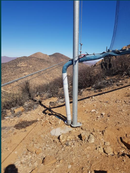
Sistema de Atrapanieblas en las quebradas de Taltal
