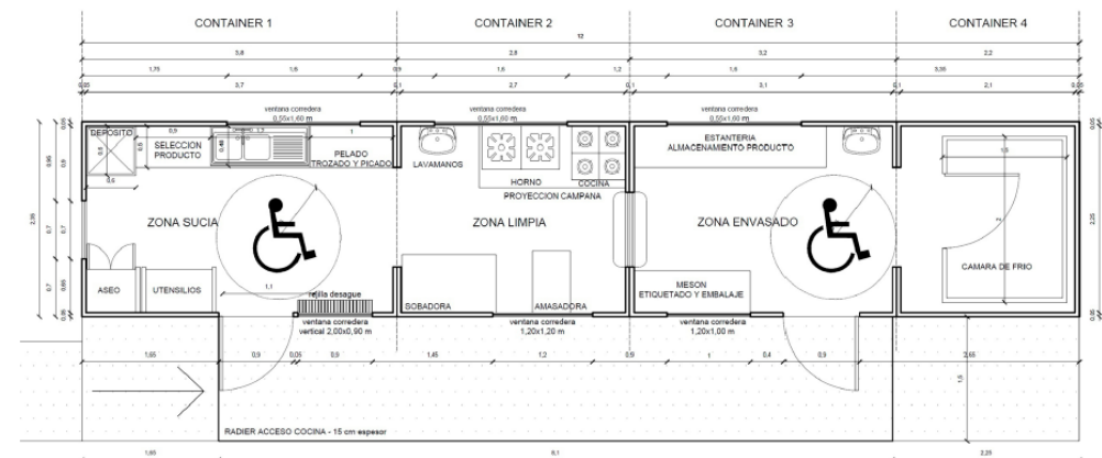
Figura 2. Plano de planta e instalaciones sanitarias de sala de procesos comunitaria Pro Til-Til.
