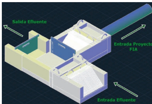
Figura 5. Diseño de sistema de pre-tratamiento del agua residual urbana tratada.
