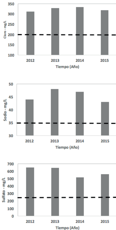
Figura 3. Concentración de sales del Agua Residual Urbana Tratada de la Planta Pozo Almonte
