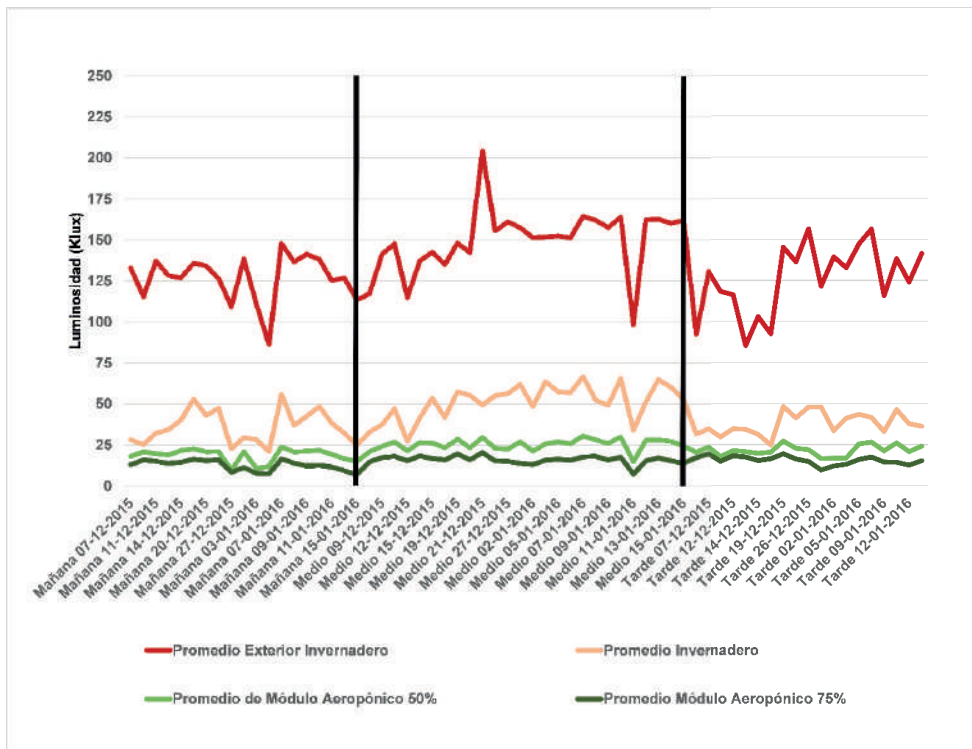
Figura 34. Intensidad de luminosidad en ambientes internos y externos del invernadero en la mañana, mediodía y tarde. Pozo Almonte
