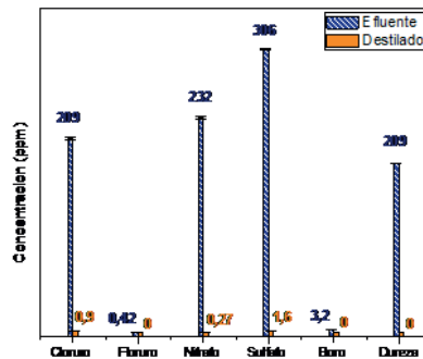
Figura 14. Concentración de iones, boro y dureza obtenida en el agua destilada.
