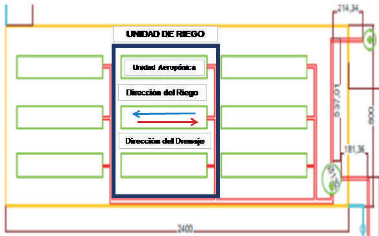
Figura 17. Diseño del sistema de riego. Pozo Almonte
