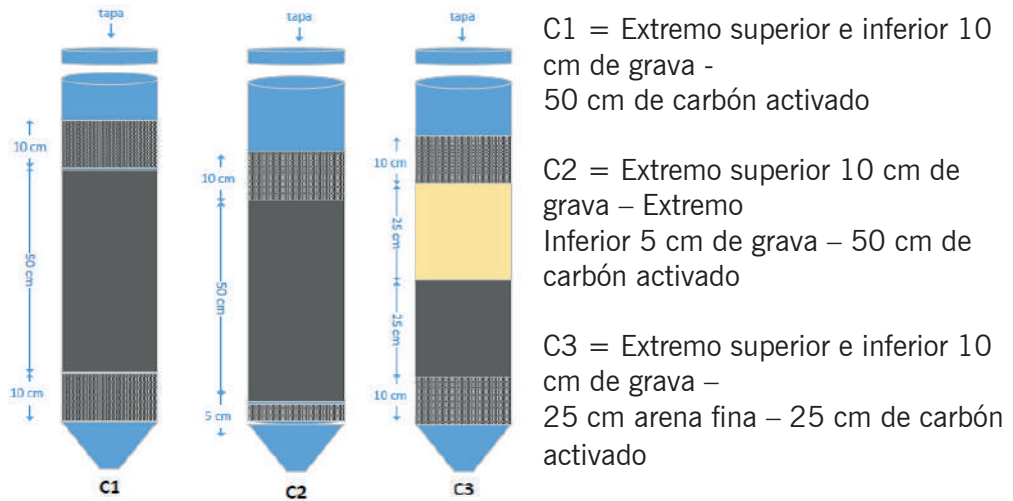
Figura 8. Esquema de los sistemas de filtración implementados para la remoción de boro del agua residual urbana tratada. Laboratorio CIDERH
