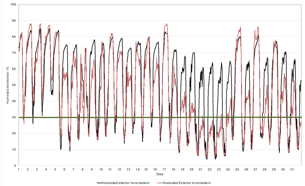
Figura 31. Variación mensual de la humedad ambiental interior y exterior del invernadero durante Julio 2016. Pozo Almonte.
