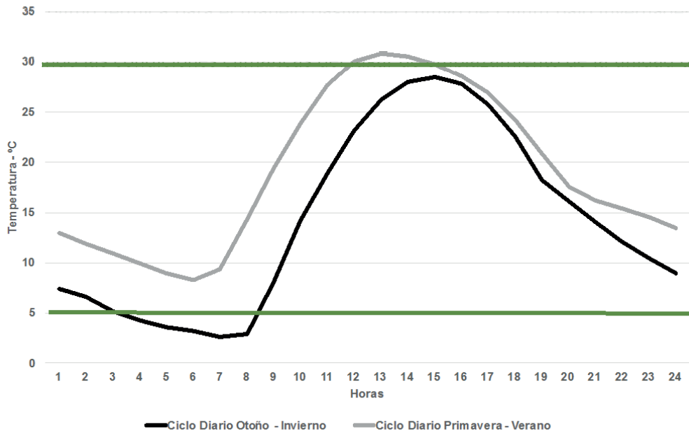
Figura 25. Evolución de la temperatura promedio durante ciclo diario. Estación climática externa a invernadero. Pozo Almonte.
