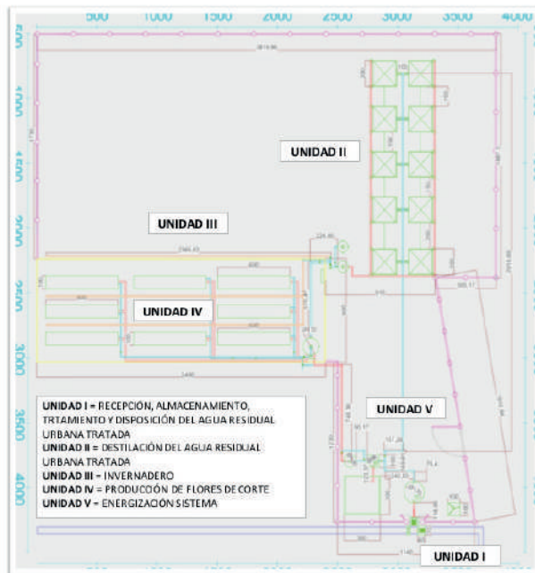
Figura 1.- Plano de planta del proyecto de producción de flores de corte en un sistema aeropónico recirculante con agua residual urbana tratada.
