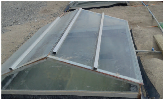
Figura 12. Destilador solar pasivo de 2 m 2 . Pozo Almonte
