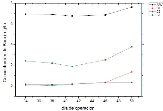
Figura 9. Resultados de las determinaciones analíticas para establecer la concentración de boro en agua, realizados durante 50 días de operación, para el influente (ARUT), y para el efluente proveniente de las columnas de filtración C1, C2, C3.
