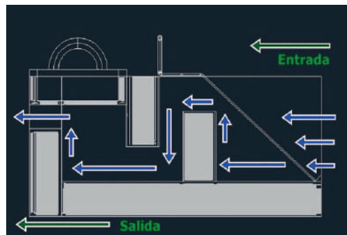
Figura 6. Decantador en sistema T.
